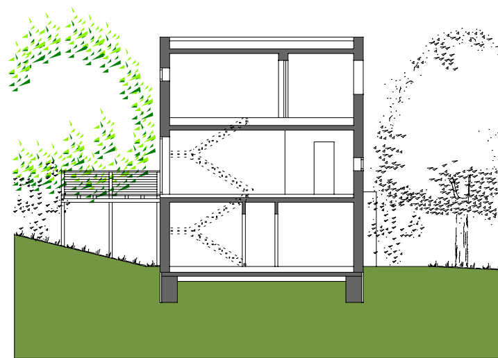
SCHNITT
