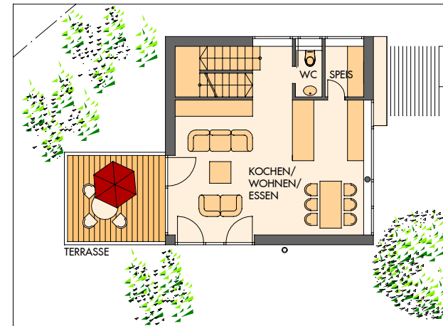
EBENE 3
