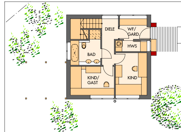
EBENE 2
