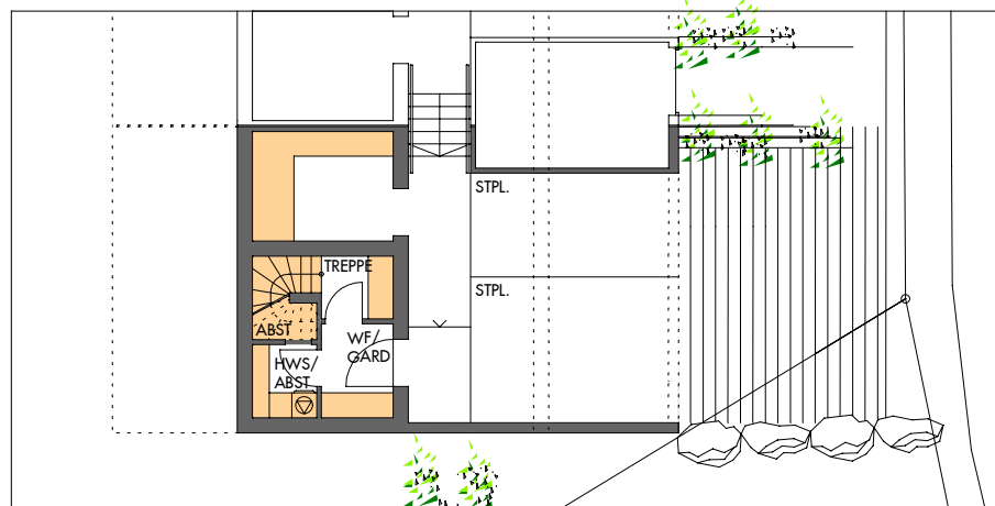
EBENE 0
