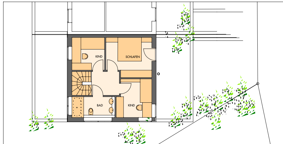
EBENE 2
