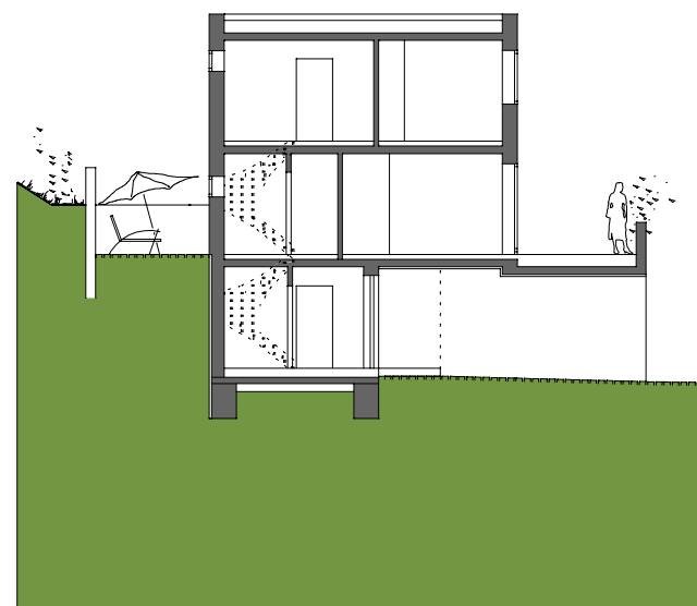
SCHNITT
