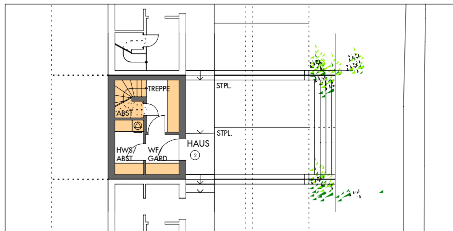
EBENE 0
