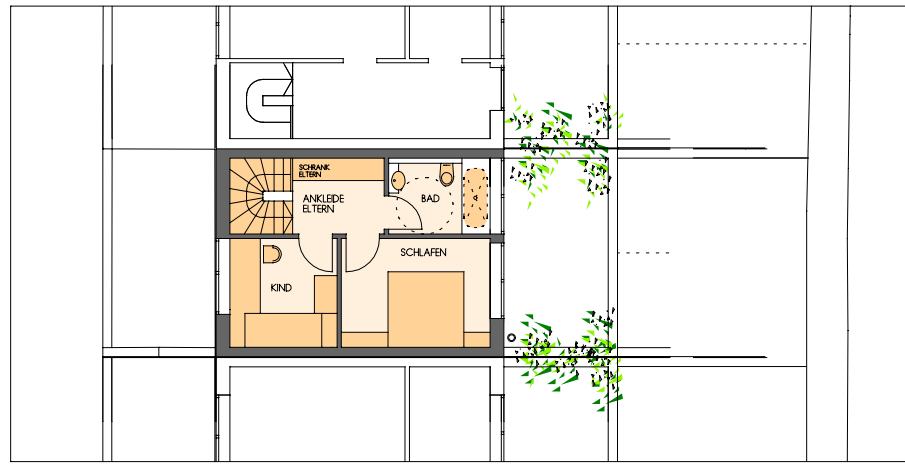
EBENE 2
