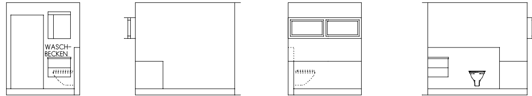
BAD OBERGESCHOSS
